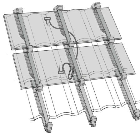
Kabel verbinden
