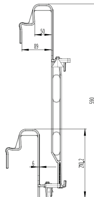
Abmaße der SOLo Haken
