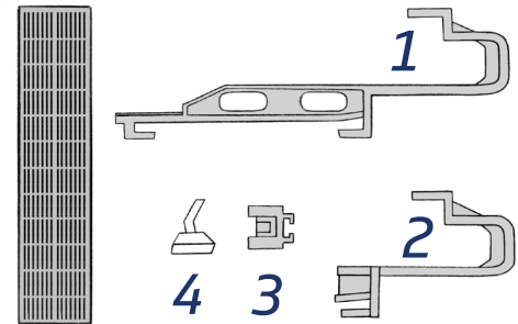
Übersicht Systemkomponenten
