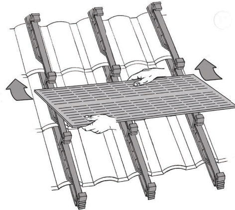
Module einsetzen
