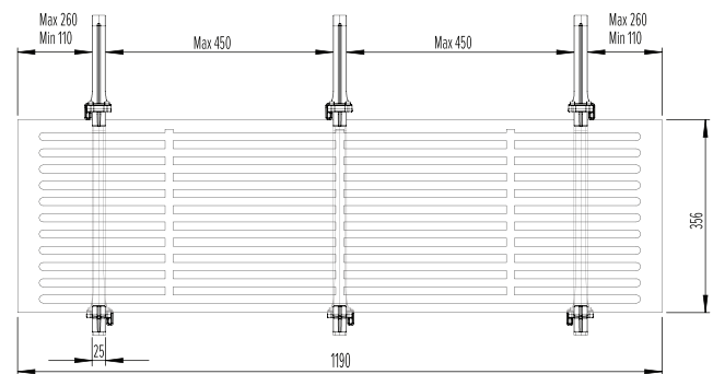
Klemmbereiche 1 am SOLo PV-Modul
